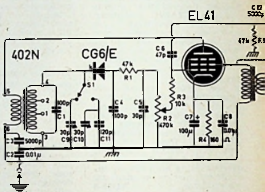
SCHAKELING „SOLOFLEX” RB Maart '55)
