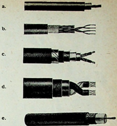
Afb. 2 - a. soepele hoogspanningsleiding; b. blanke emaille-loodkabel, meeraderig; c. gepantserde rubber loodkabel (GRIK); d. rubber werkplaatskabel (RWPK of BRML) met twee rubber mantels; e. coaxiale kabel. (Foto's: DRAKA, A'dam)
