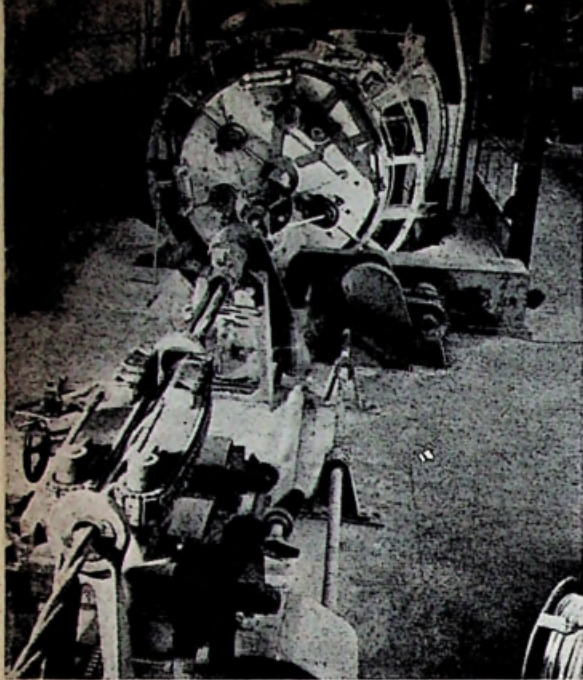
Afb. 4 - MACHINE VOOR HET SAMEN- SLAAN VAN DE ADERS IN EEN KABEL (Foto: N.V. Holl. Draad- en Kabelfabriek, Amsterdam)
